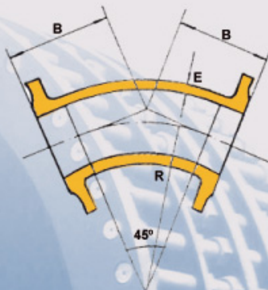
Curvas BB 1/8 ( 45°)
