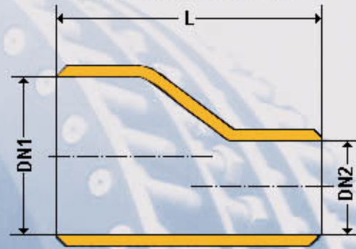
Reducción AC Excéntrica
