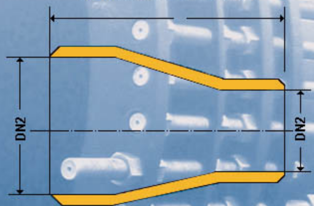
Reducción AC Concéntrica
