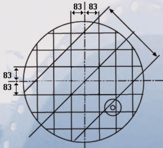
TAPA ALCANTARILLADO
